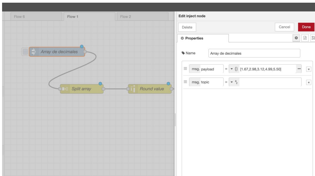
Ilustración 18. Envío de array con número decimales en Node-RED
