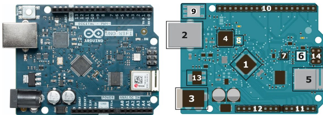
Ilustración 6. Estructura de una placa Arduino UNO WiFi REV2
