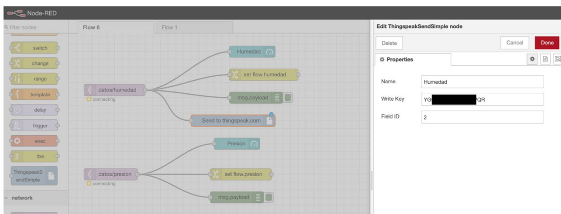
Ilustración 85. Utilización del nodo "thingspeak" en Node-RED
