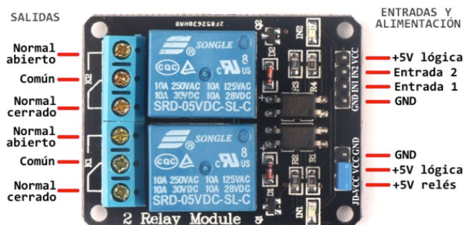
Ilustración 80. Conexiones de un relé
