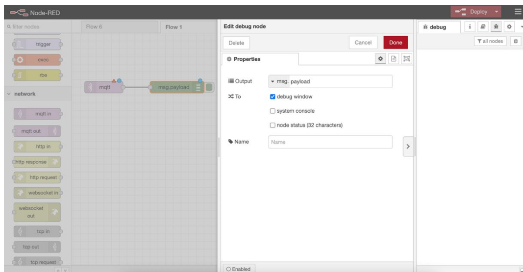
Ilustración 42. Configuración del nodo "debug" en Node-RED
