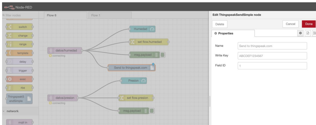
Ilustración 83. Uso del nodo "thingspeak" para el envío de datos en Node-RED
