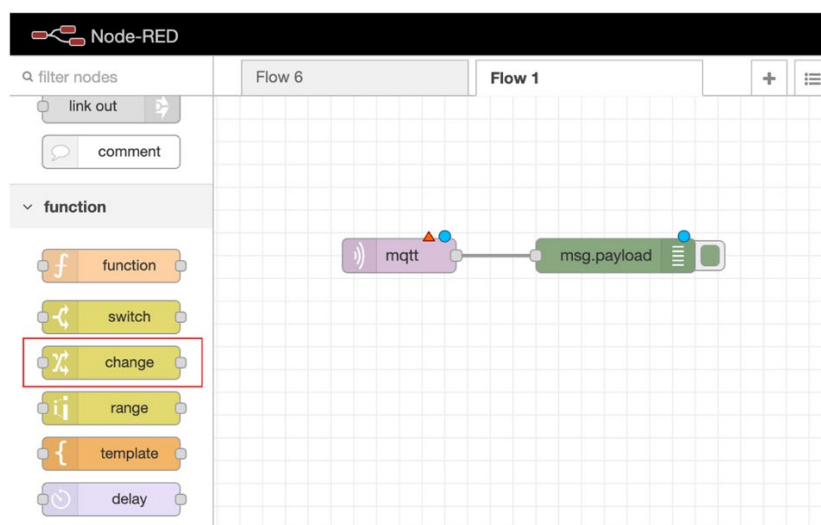
Ilustración 43. Localización del nodo "change" en Node-RED
