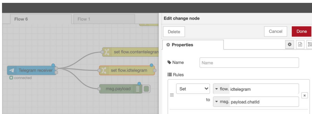
Ilustración 64. Cambio de nombre y contexto de las variables de Telegram en Node-RED
