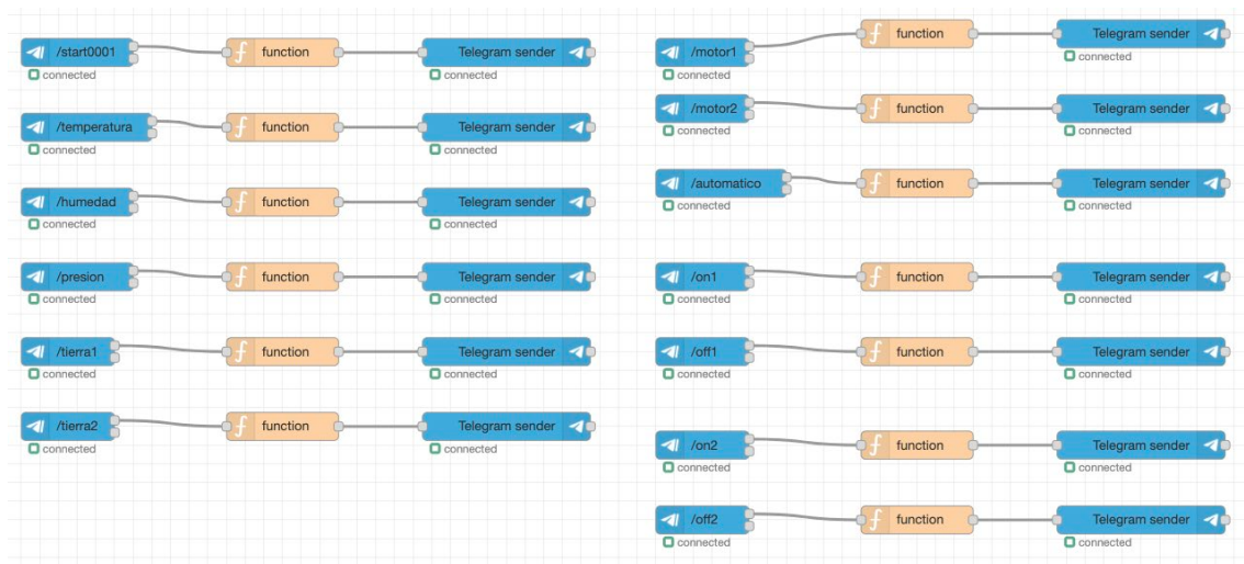
Ilustración 72. Esquema general de los comandos disponibles de Telegram
