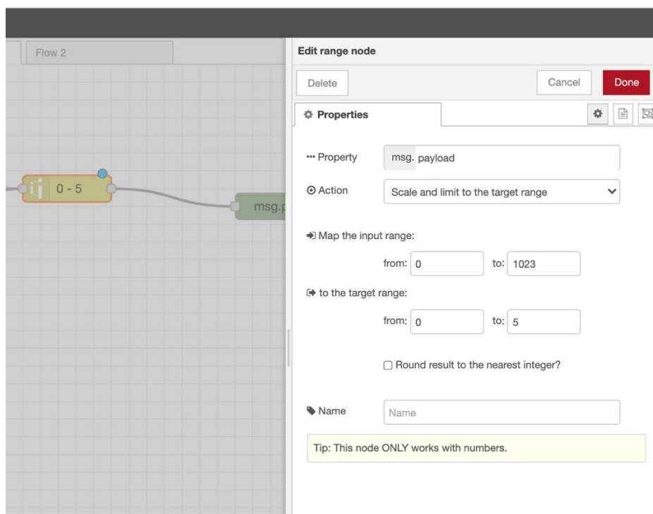
Ilustración 16. Menú nodo “range” de Node-RED
