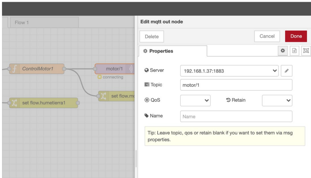
Ilustración 68. Servidor y topic donde se va a publicar la información de la función de control
