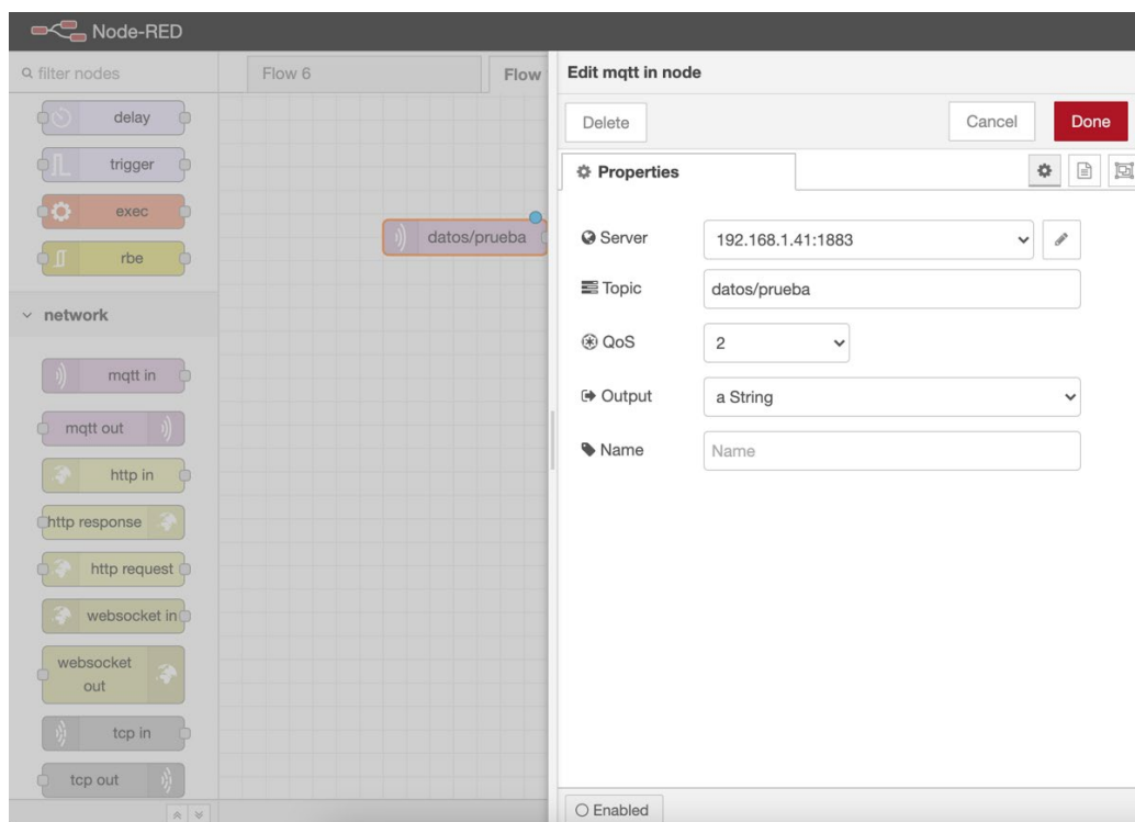
Ilustración 37. Menú del nodo "mqtt in" en Node-RED
