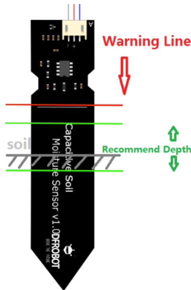
Ilustración 27. Sensor de humedad de suelo SKU:SEN0193
