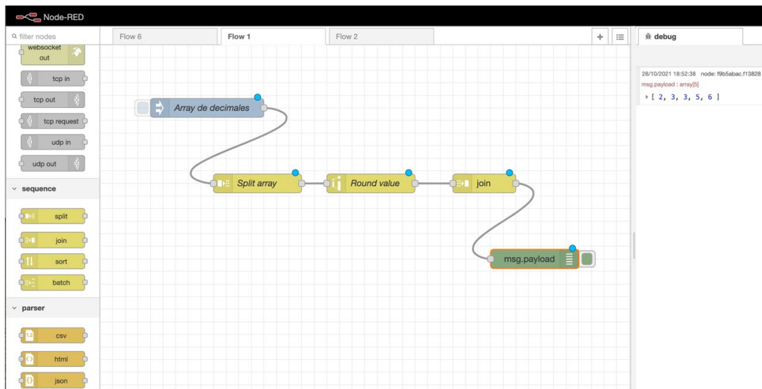
Ilustración 20. Redondeo array de decimales en Node-RED
