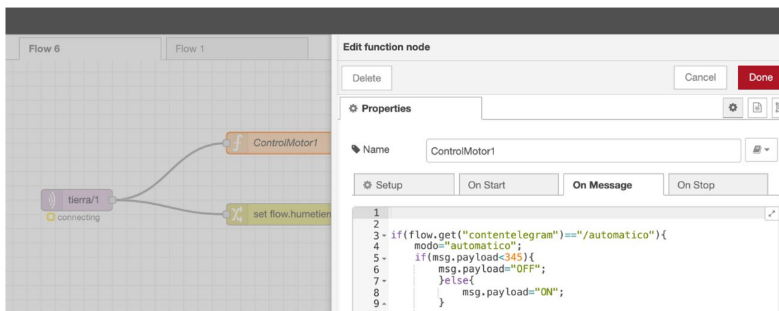
Ilustración 67. Primera condición de automatización de la función de control
