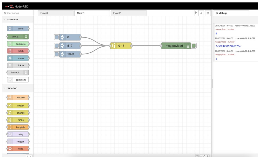
Ilustración 17. Cambiar rango de números en Node-RED
