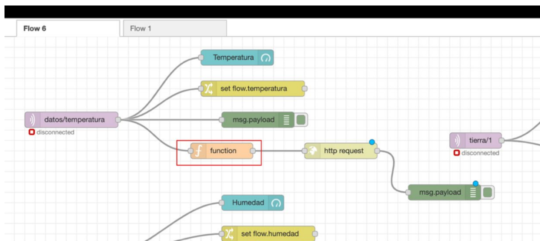
Ilustración 88. Esquema general del envío de la información a ThingSpeak
