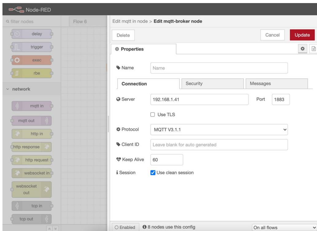
Ilustración 38. Configuración de la conexión del nodo "mqtt in" en Node-RED
