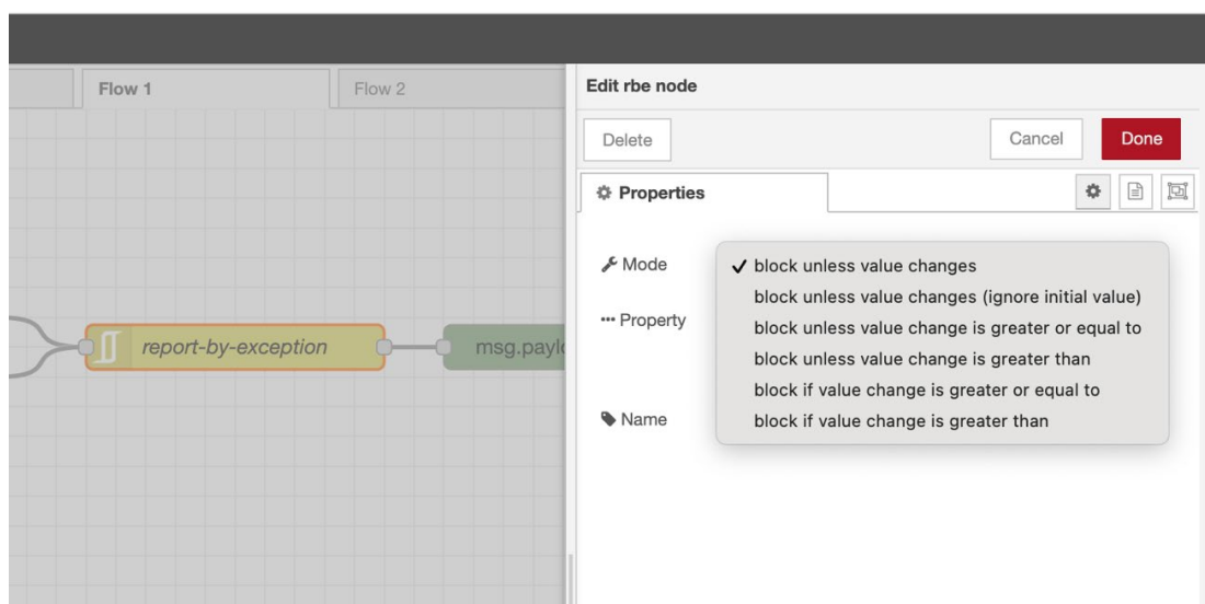
Ilustración 21. Menú del nodo “rbe” de Node-RED
