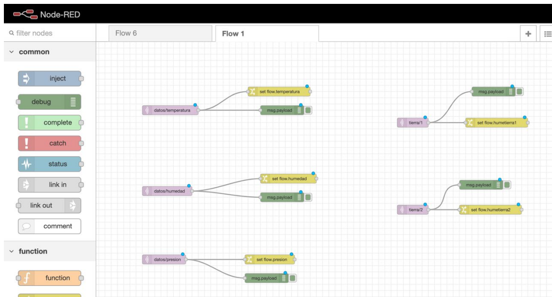
Ilustración 45. Esquema general de la recepción de datos y el cambio de contexto en Node-RED
