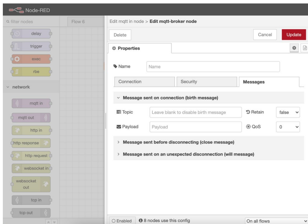
Ilustración 40. Tipos de mensajes en el nodo "mqtt in" de Node-RED
