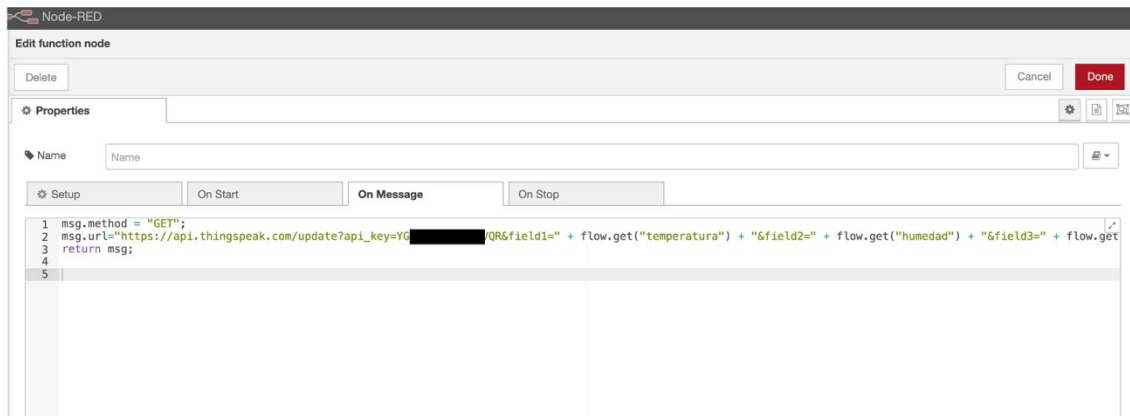
Ilustración 87. Envío de una petición HTTP con los datos de Node-RED a ThingSpeak
