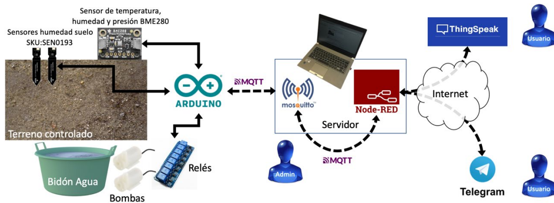
Ilustración 25. Esquema práctico general
