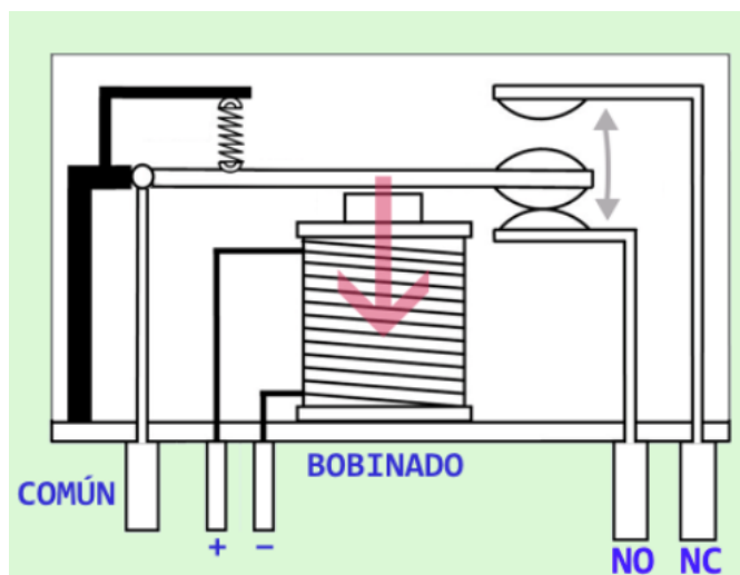
Ilustración 79. Esquema interno de un relé
