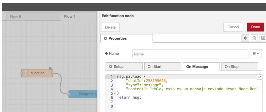
Ilustración 58. Función para el envío de datos de Node-RED a Telegram
