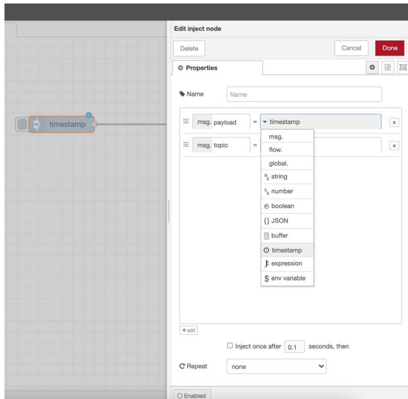
Ilustración 12. Uso Timestamp en Node-RED
