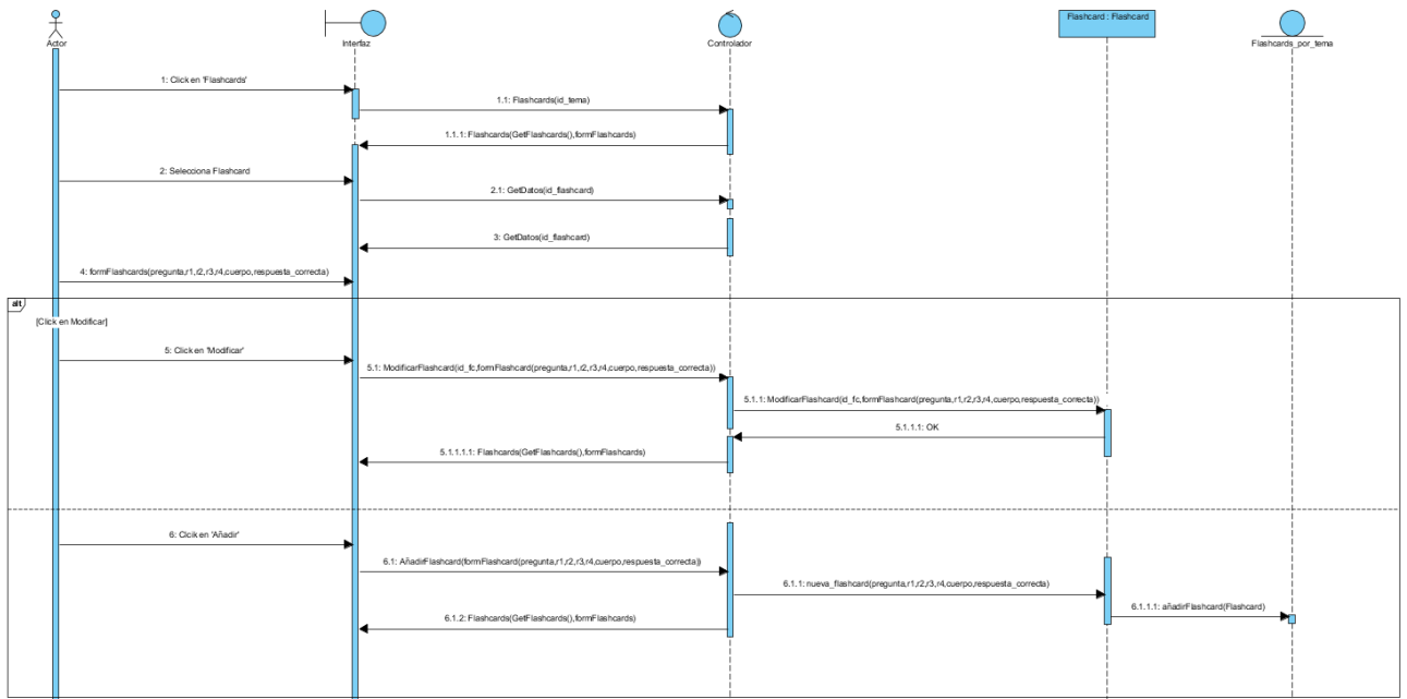
Ilustración 57. Diagrama de Secuencia: Editar flashcard
