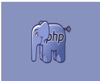
Ilustración 4. Logo PHP
