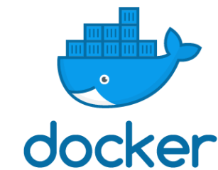
Ilustración 9. Logo Docker
