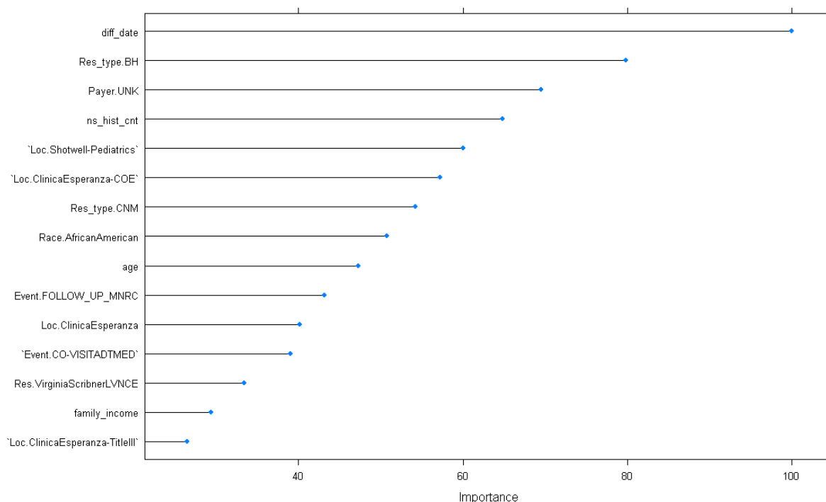
Figura 20.- Ranking de predictores algoritmos FDA.
