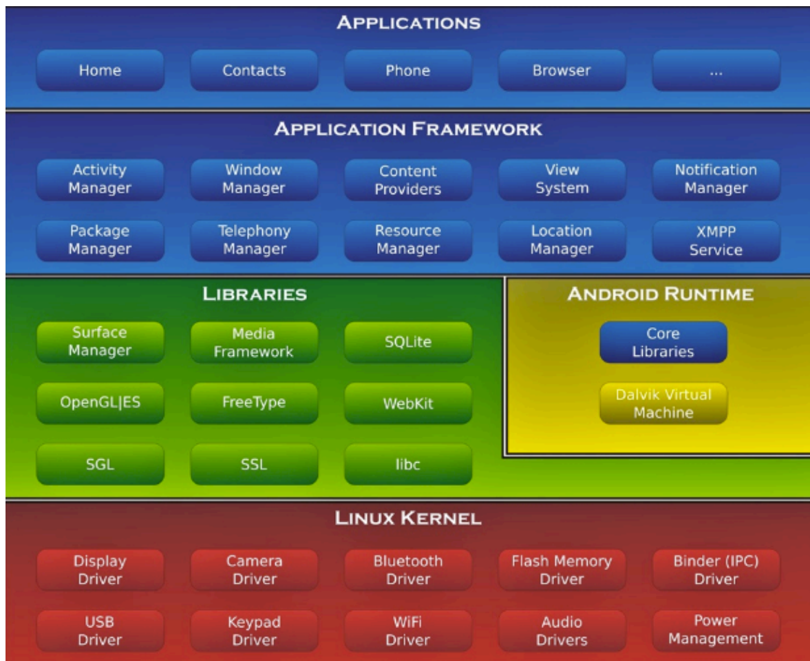
Ilustración 3.8 Arquitectura Android [25]
