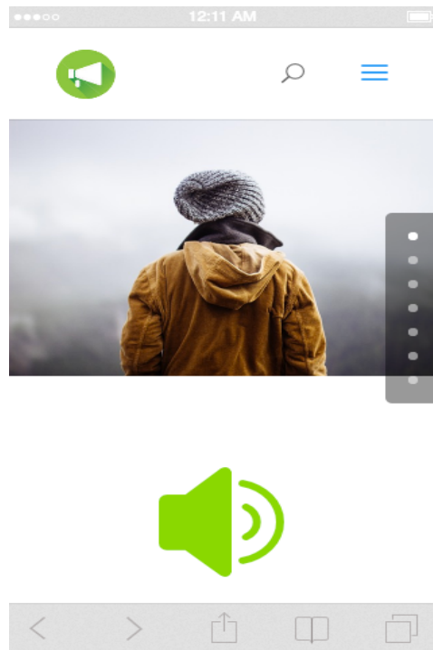
Ilustración 4.1 Página Home
