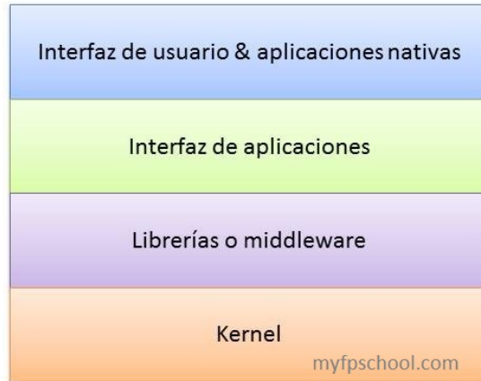
Ilustración 3.2 Capas S.O. [5]
