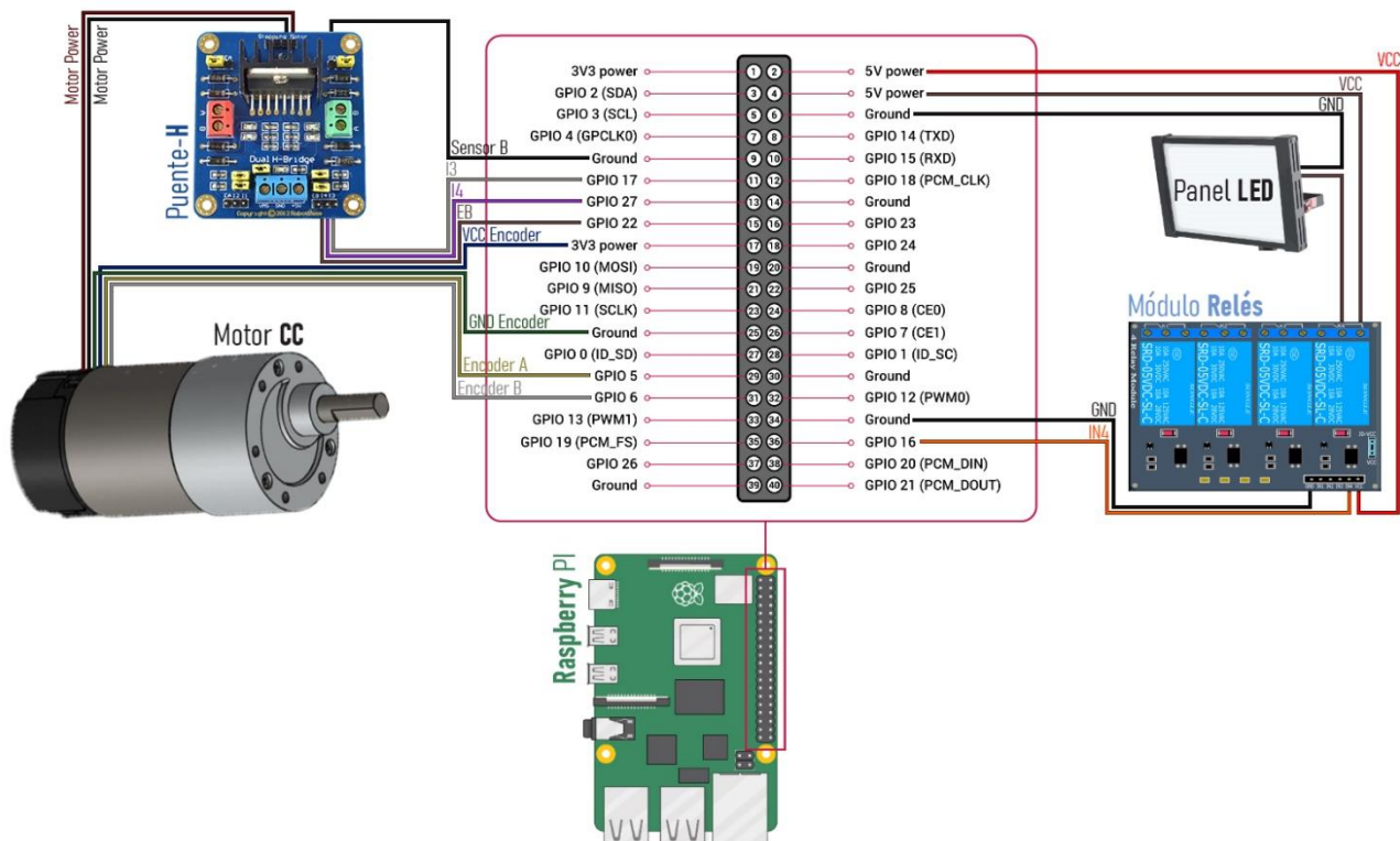
Figura 4-1.- Conexiones sistema con pines GPIO
