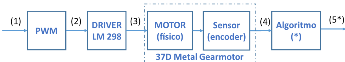
Figura 5-1. - Esquema interno para la identificación de la dinámica del motor.
