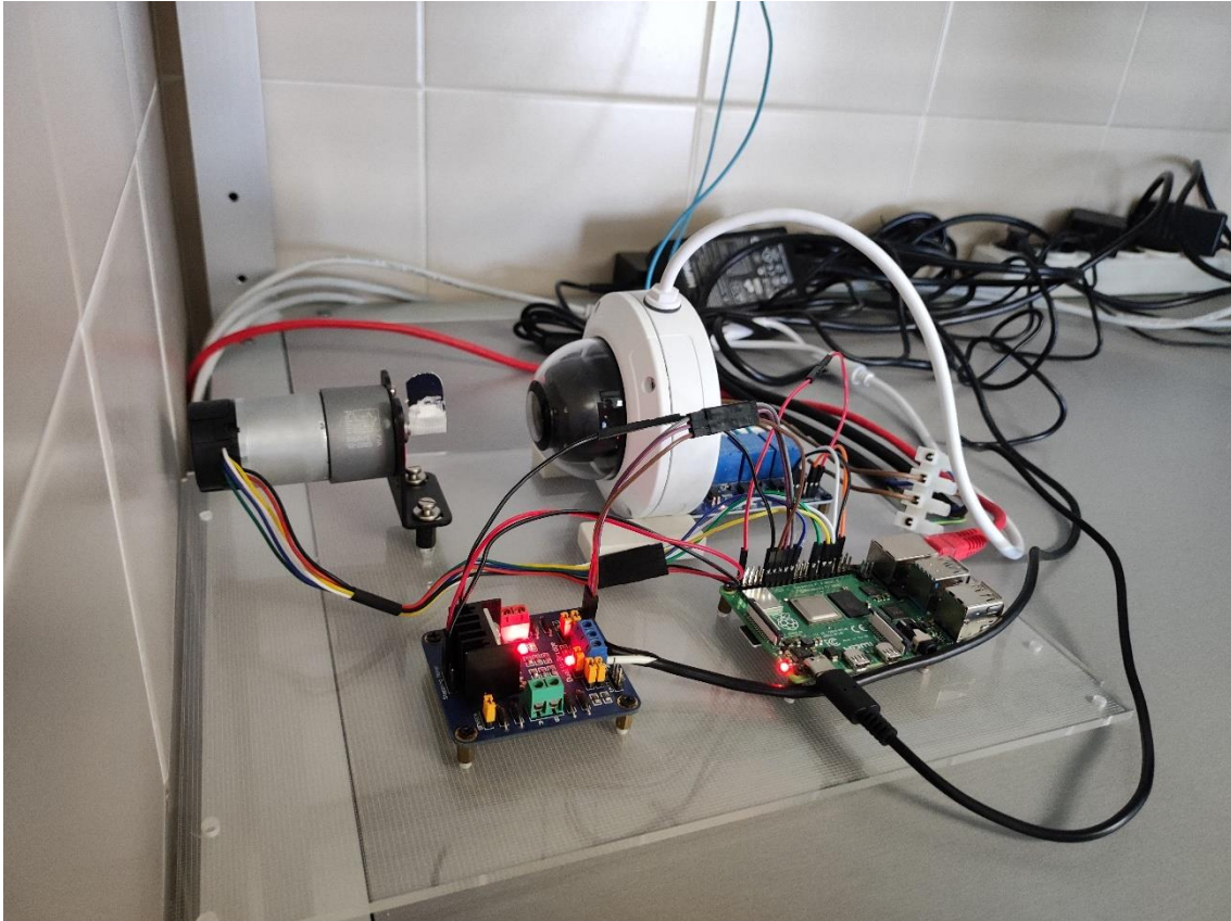
Figura 1-6.- Montaje laboratorio remoto
