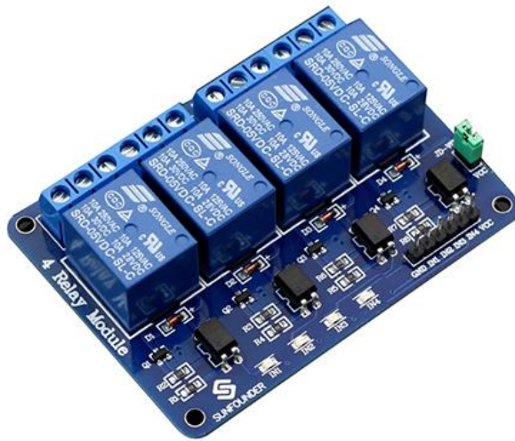
Figura 3-12.- Modulo 4 Relés
