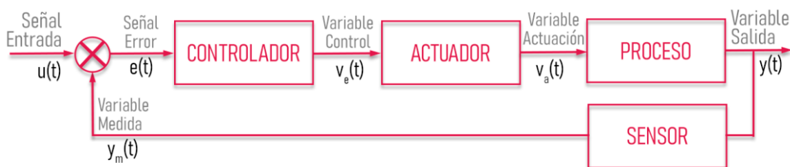
Figura 4-19.- Sistema de Control en bucle cerrado
