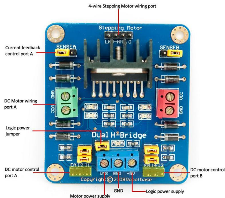
Figura 3-10.- Controlador de Motor Dual
