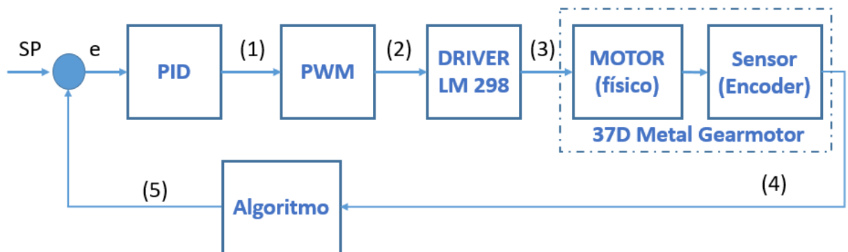
Figura 5-3.- Esquema interno para el control del sistema con un PID.
