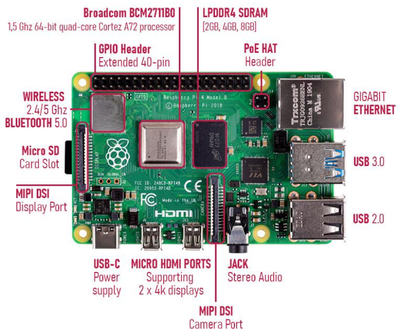
Figura 3-2.- Componentes Raspberry Pi 4 modelo B
