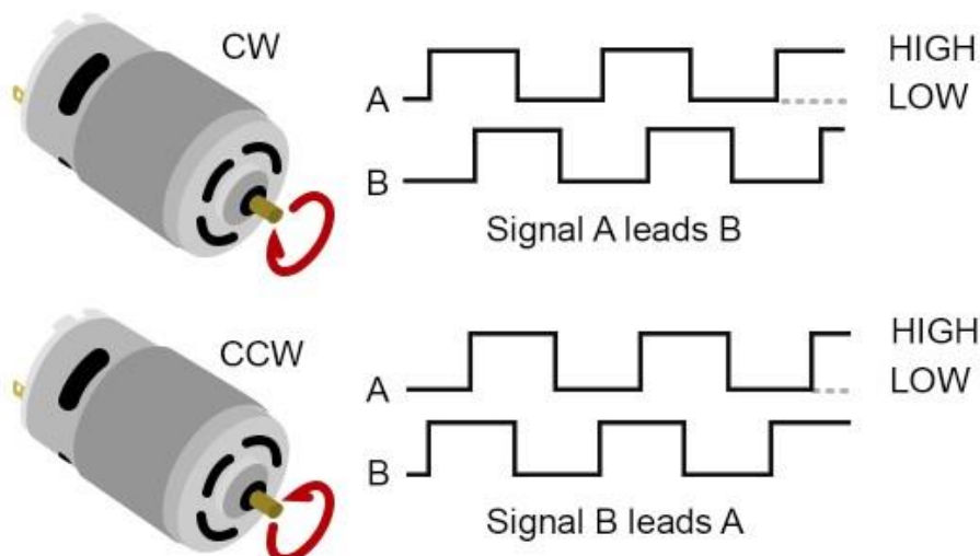
Figura 4-8.- Estados Encoder
