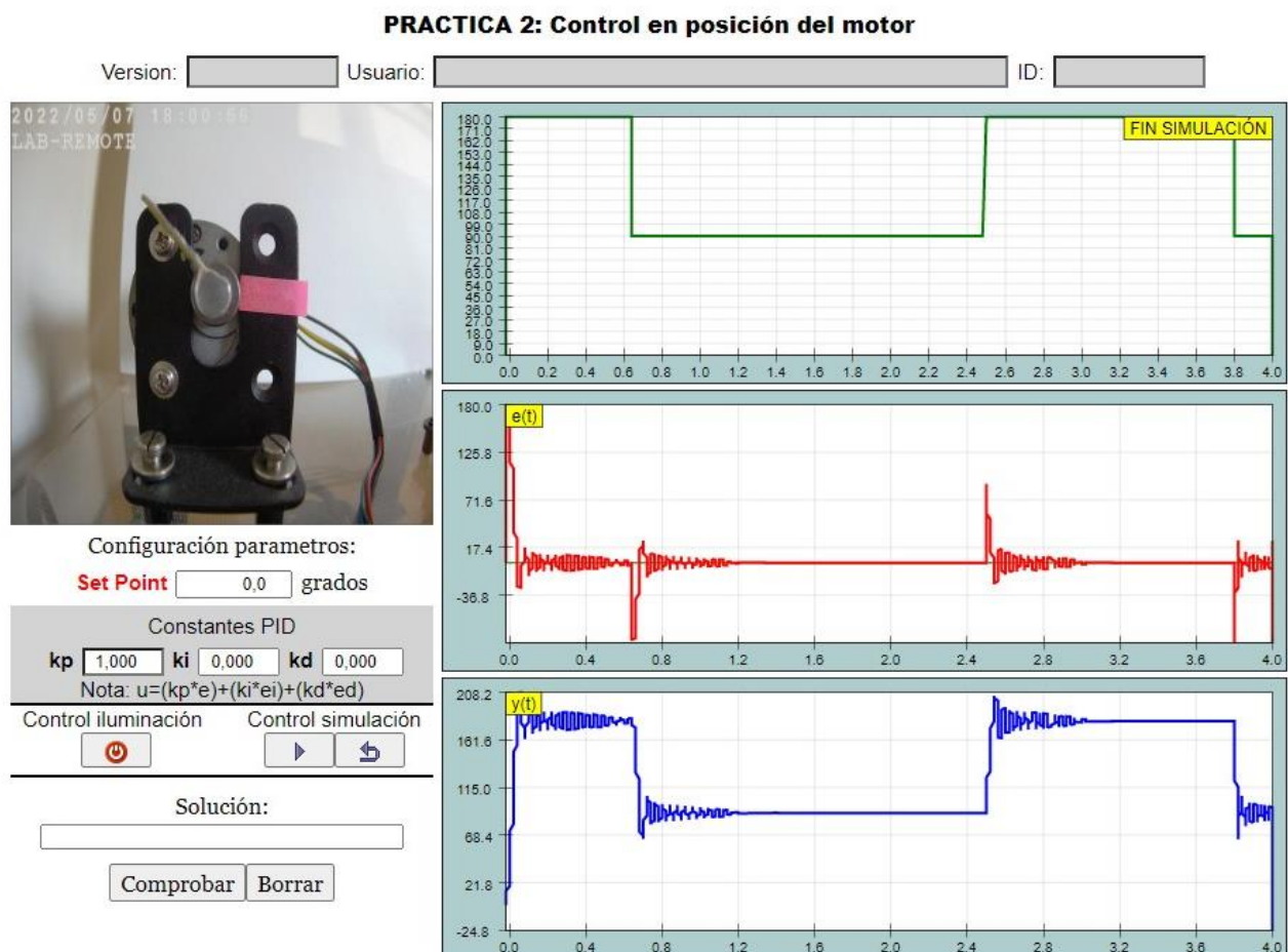
Figura 4-15.- Laboratorio remoto para el Control en posición del motor
