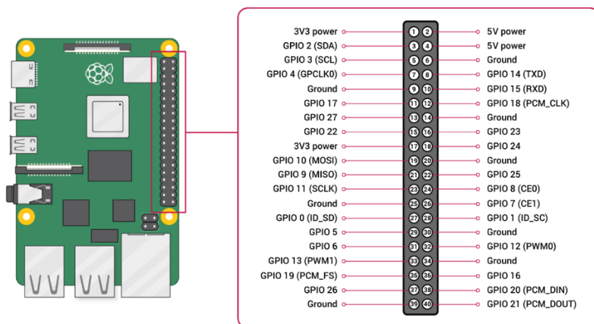
Figura 3-3.- Conexión GPIO Raspberry PI 4
