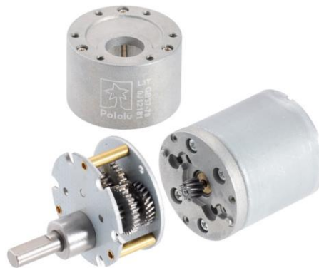
Figura 3-7.- Engranajes interiores Motor
