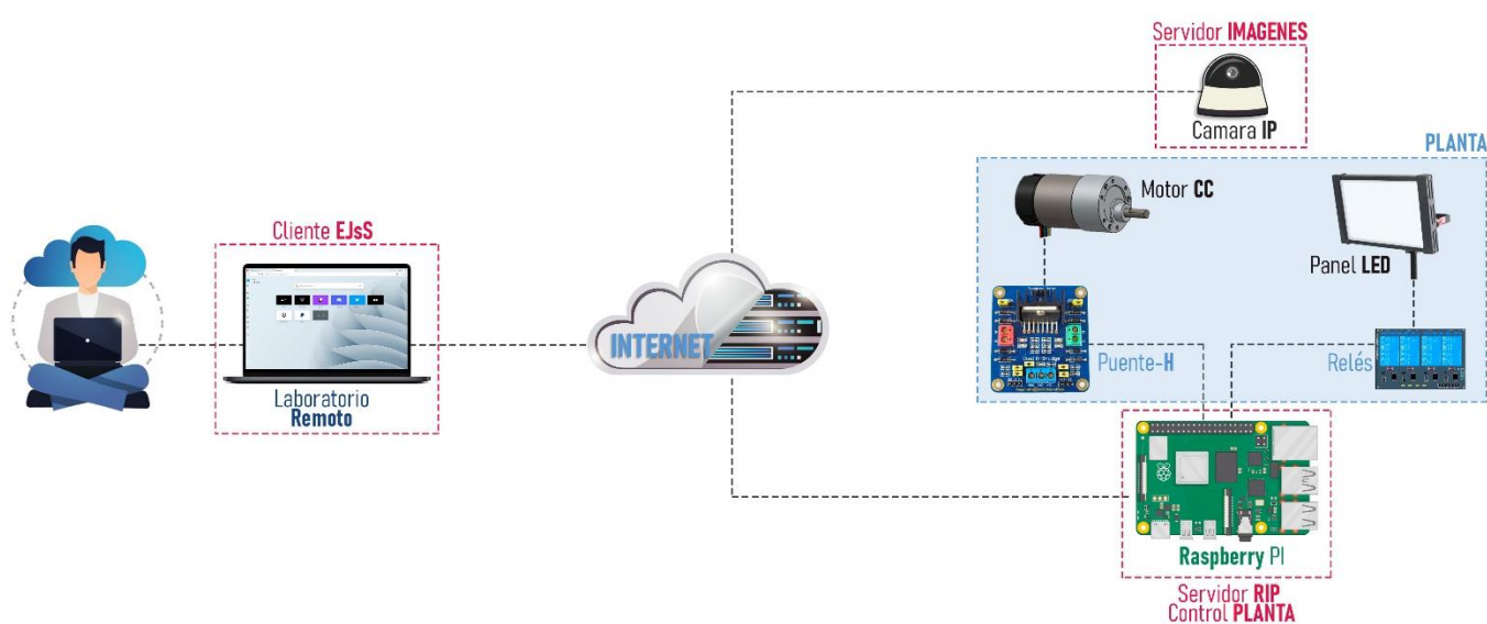
Figura 1-2.- Esquema general del sistema.
