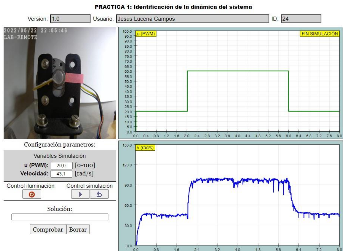
Figura 5-2.- Práctica 1: Identificación de la dinámica del sistema
