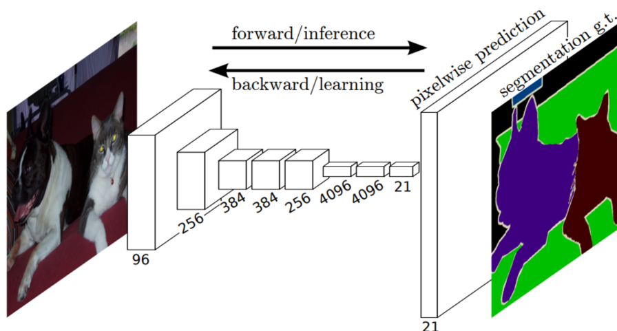
Figura 2.16: Red Neuronal Totalmente Convolucional. [10].
