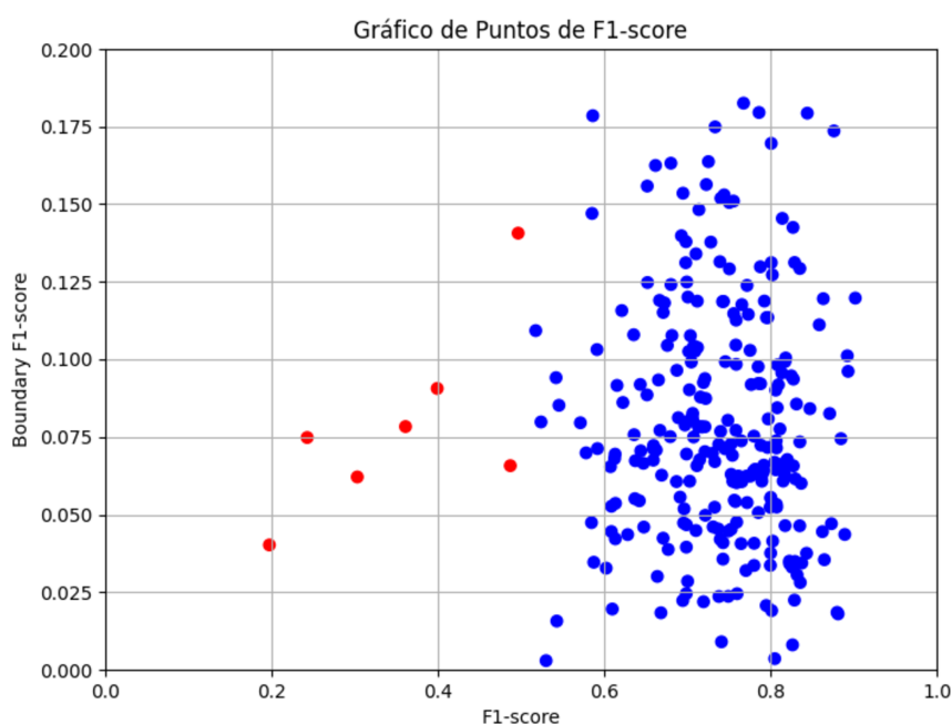
Figura 5.3: Resultados de la versión 1 representados en dos dimensiones ( F1 Score , Boundary F1 Score ). Elaboración propia.
