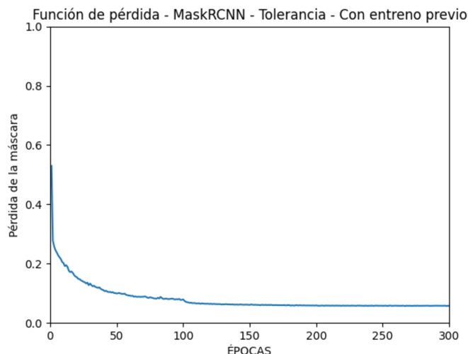
Figura 4.22: Representación de la función de pérdida de la máscara. Versión 3 del modelo final. Elaboración propia.
