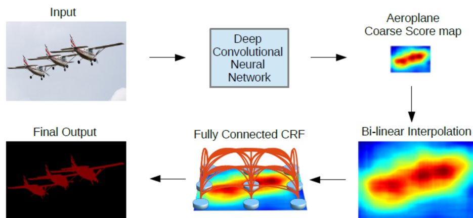
Figura 2.19: CNN unido con CRF. [12].
