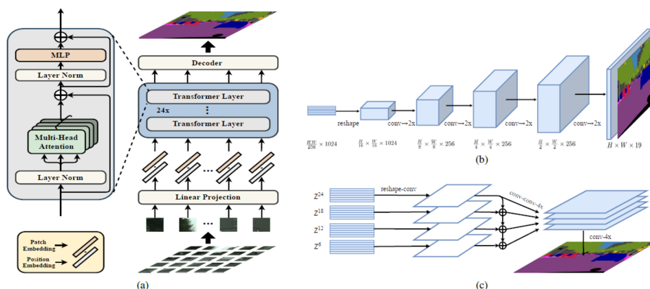
Figura 2.24: Arquitectura SETR. [17].
