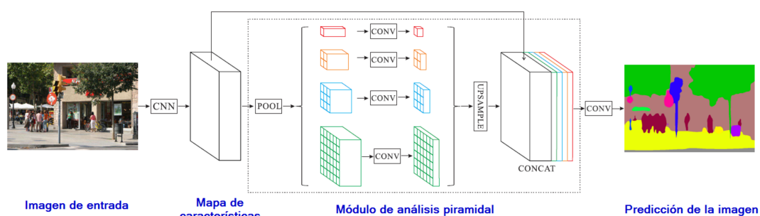
Figura 2.20: Arquitectura de la PSPNet. [13].
