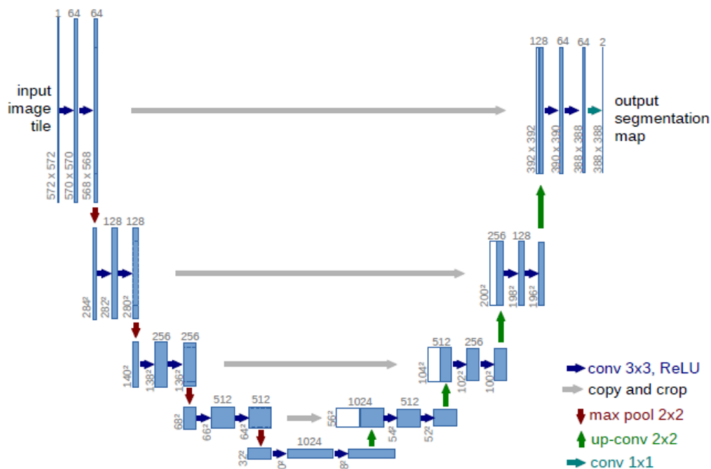
Figura 2.22: Arquitectura U-Net. [15].
