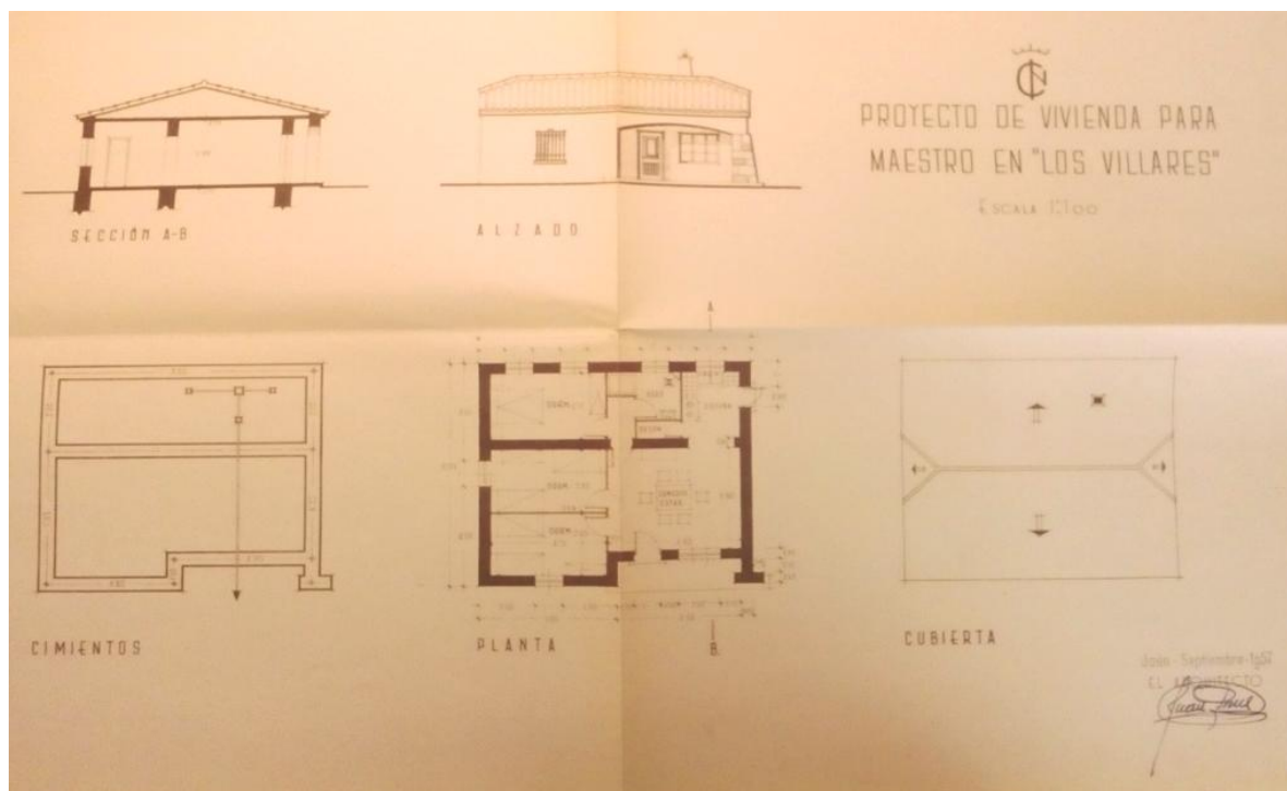
Foto: Plano de vivienda para maestro (Archivo Histórico Provincial de Jaén) Legajo 43.200
