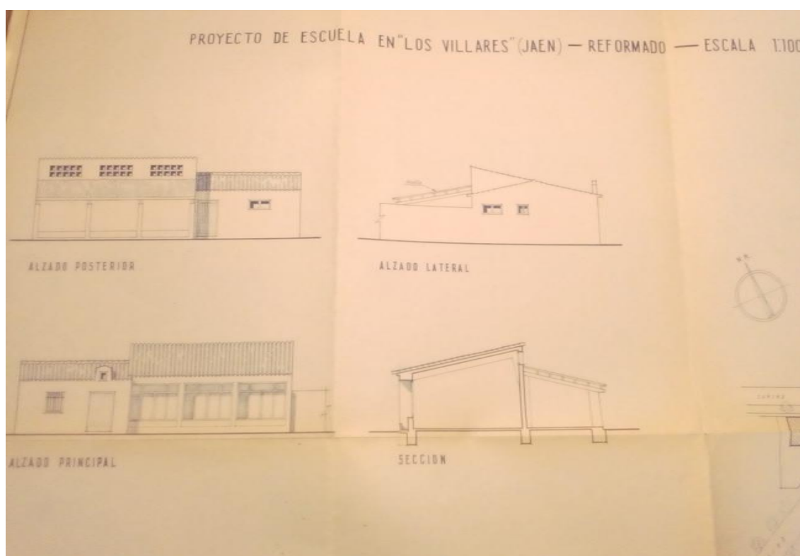
Foto: Plano de proyecto de escuela en Los Villares. (Información proveniente del Archivo Histórico Provincial de Jaén.) Legajo 43.200
