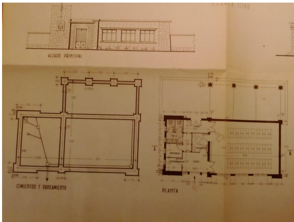
Foto: Planos de proyecto de escuela en Los Villares.( Archivo Histórico Provincial de Jaén.)
