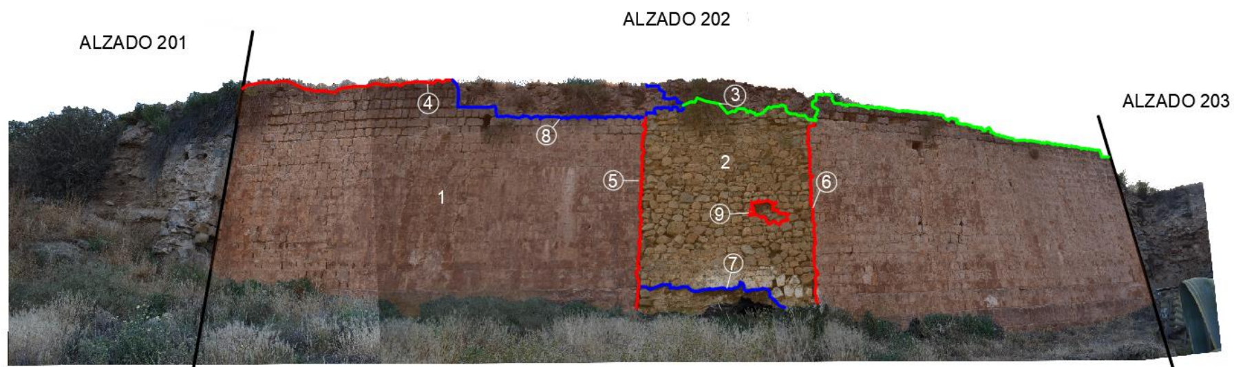
ZONA 2. TRAMO D (I). ALZADO 202
