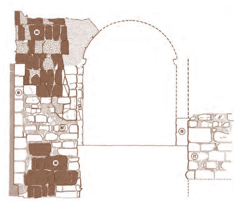
Figura 40. Alzado de la puerta Norte de la alcazaba de Priego de Córdoba con el despiece de sillería califal señalado sobre las fábricas bajomedievales (Carmona, 2009b: 238).
