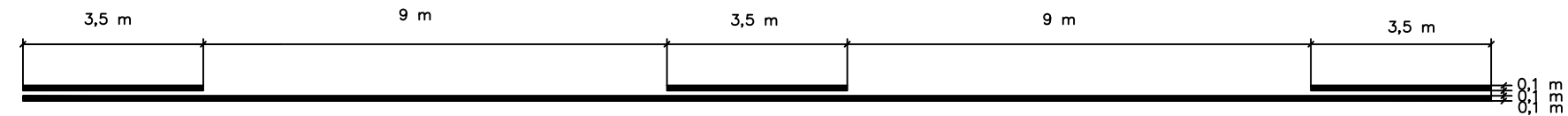
MARCA M-3.2.: VÍAS CON 60 Km/h < VM < 100 km/h- PARA REGULACIÓN DE ADELANTAMIENTO.
