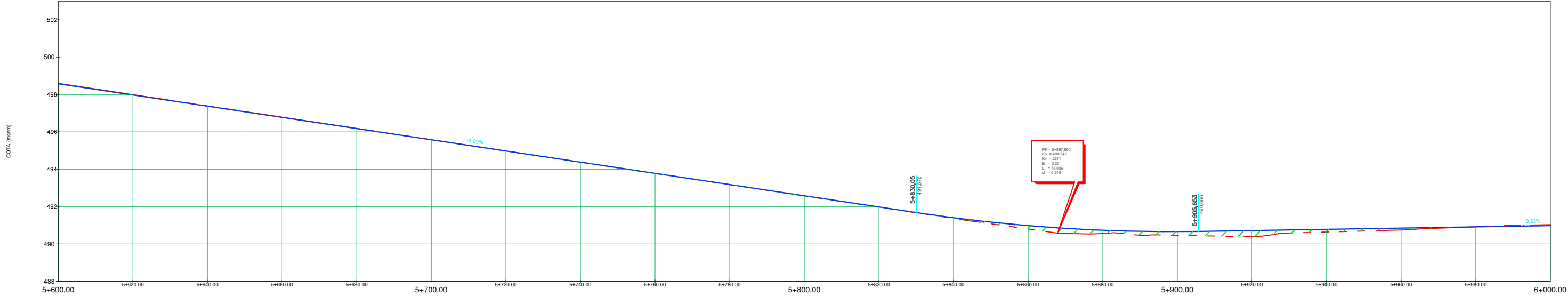
Perfil Longitudinal: Alineación carretera Escala - V: 100 H:500
