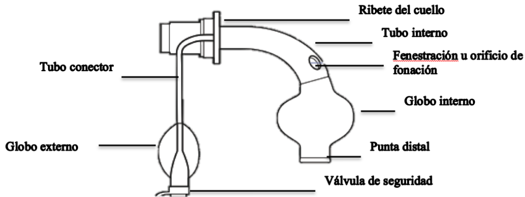
Figura 1. Vista lateral de una cánula. (Fuente propia)
