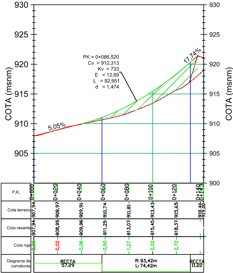
Perfil Longitudinal: Calle Eras Altas este Escala - V: 100 H:500
