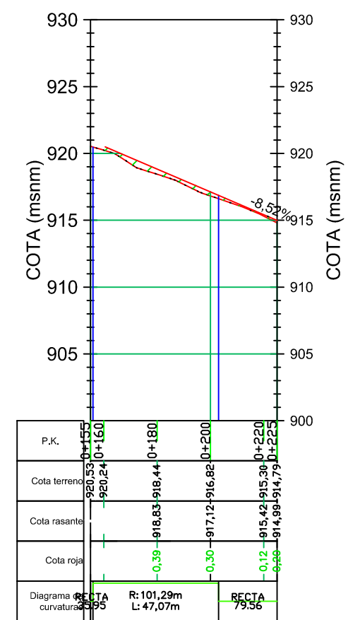
Perfil Longitudinal: JA-4302 este Escala - V: 100 H:500
