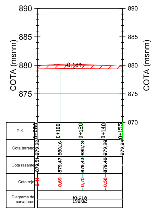
Perfil Longitudinal: A-403 (oeste) Escalas - V: 100 H:500
