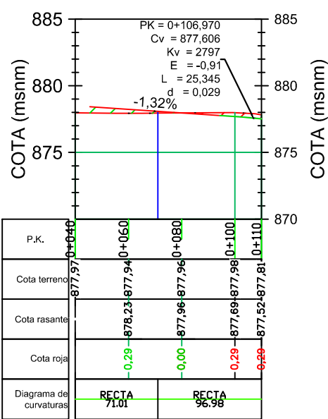
Perfil Longitudinal: Llanos de Mazuelos Escalas - V: 100 H:500
