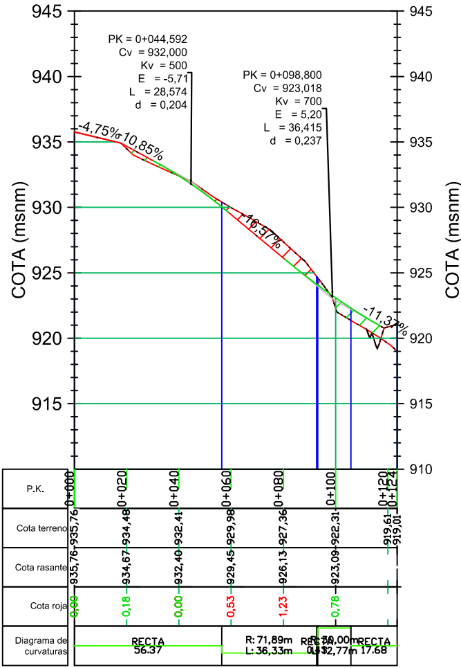
Perfil Longitudinal: Eras Altas oeste Escala - V: 100 H:500
