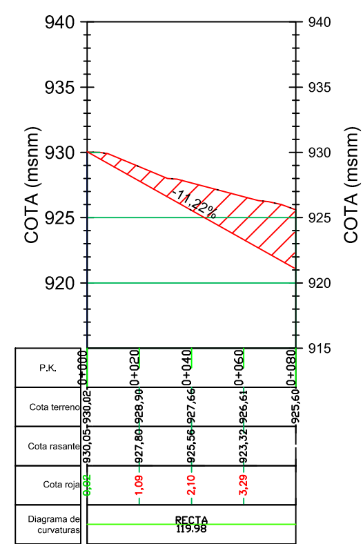
Perfil Longitudinal: JA-4302 (oeste) Escala - V: 100 H:500
