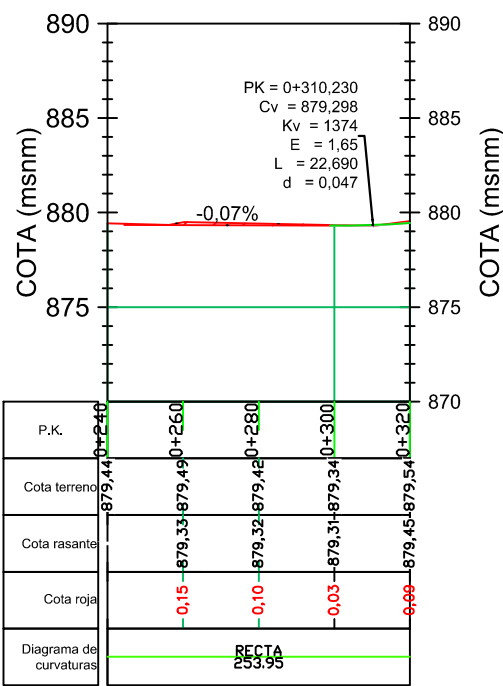
Perfil Longitudinal: A-403 (este) Escalas - V: 100 H:500
