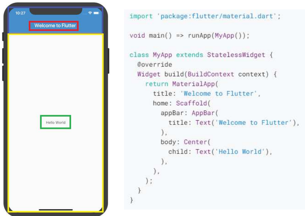
Ilustración 10. Representación de widgets
