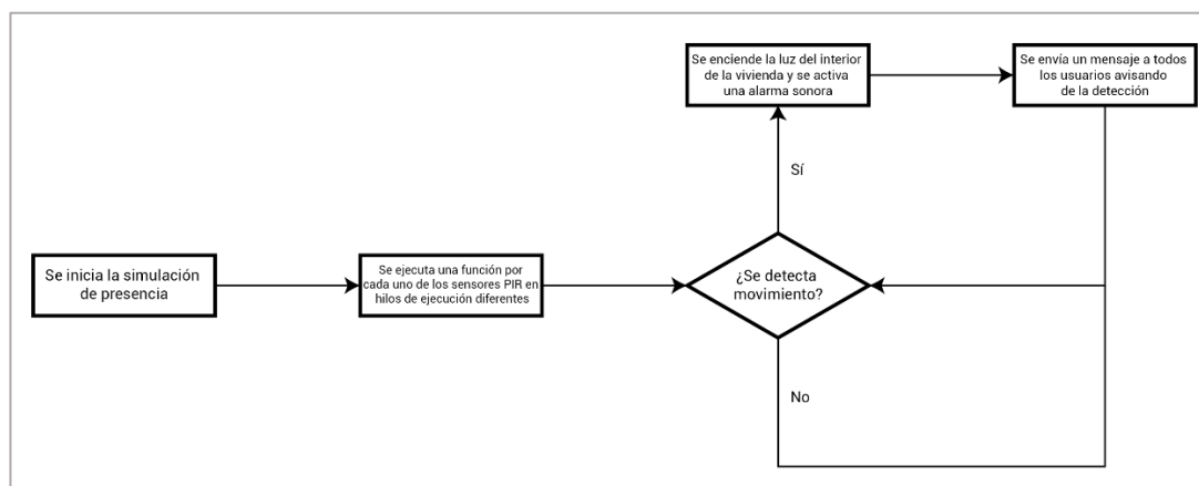
Figura 39: Flujograma de la simulación de presencia con alarma
