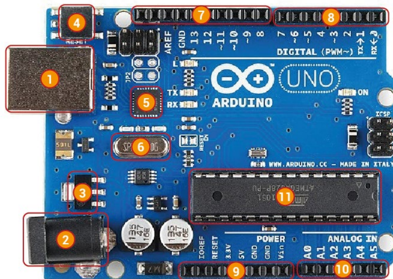
Figura 11: Arduino UNO R3
