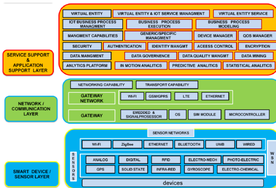
Figura 5: Arquitectura IoT
