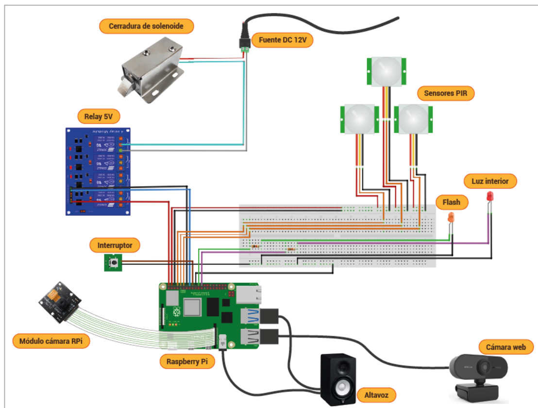
Figura 16: Esquema general de los componentes electrónicos del sistema de seguridad
