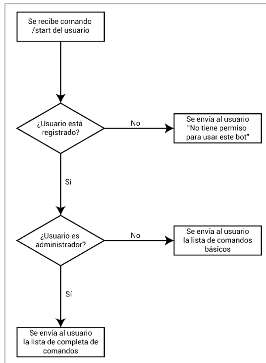
Figura 20: Flujograma del comando /start
