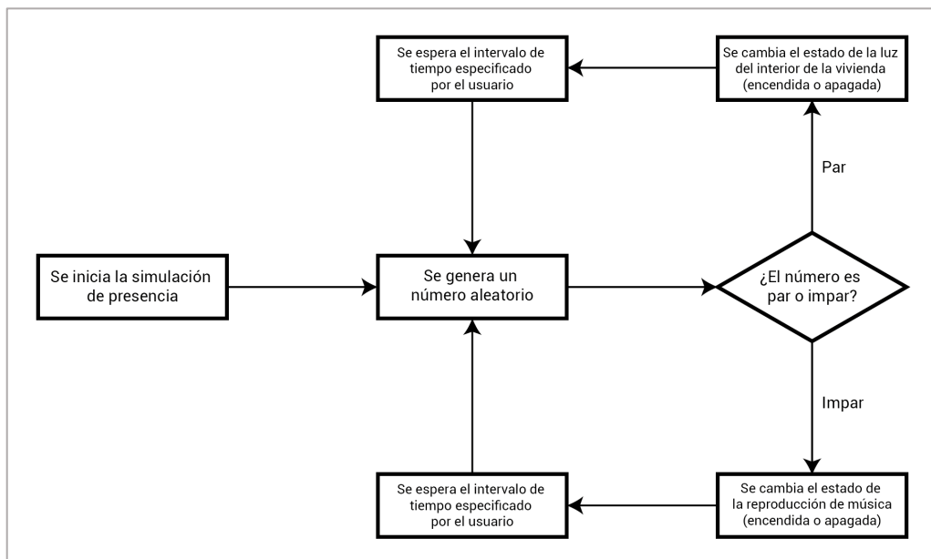
Figura 36: Flujograma de la simulación de presencia aleatoria
