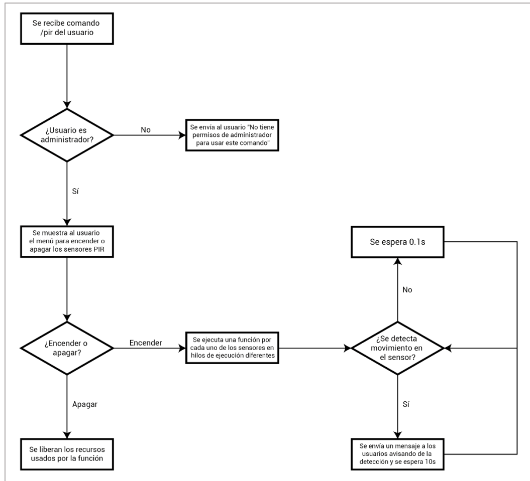
Figura 31: Flujograma del comando /pir
