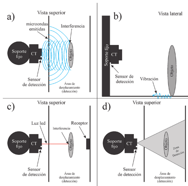
Figura 6: Funcionamiento de un sensor por microondas
