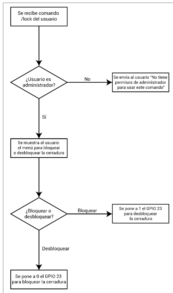
Figura 26: Flujograma del comando /lock
