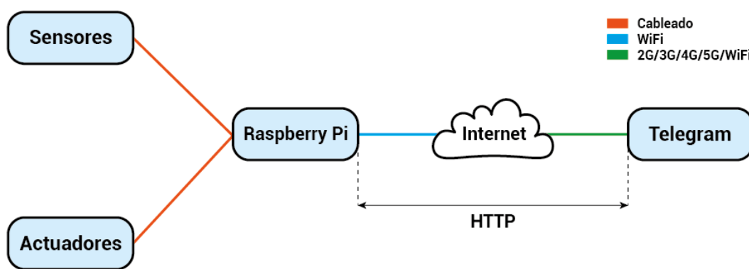
Figura 15: Esquema de las comunicaciones del sistema de seguridad
