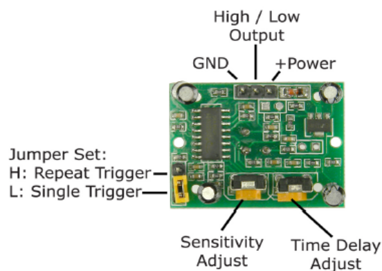
Figura 9: Patillaje de un sensor PIR
