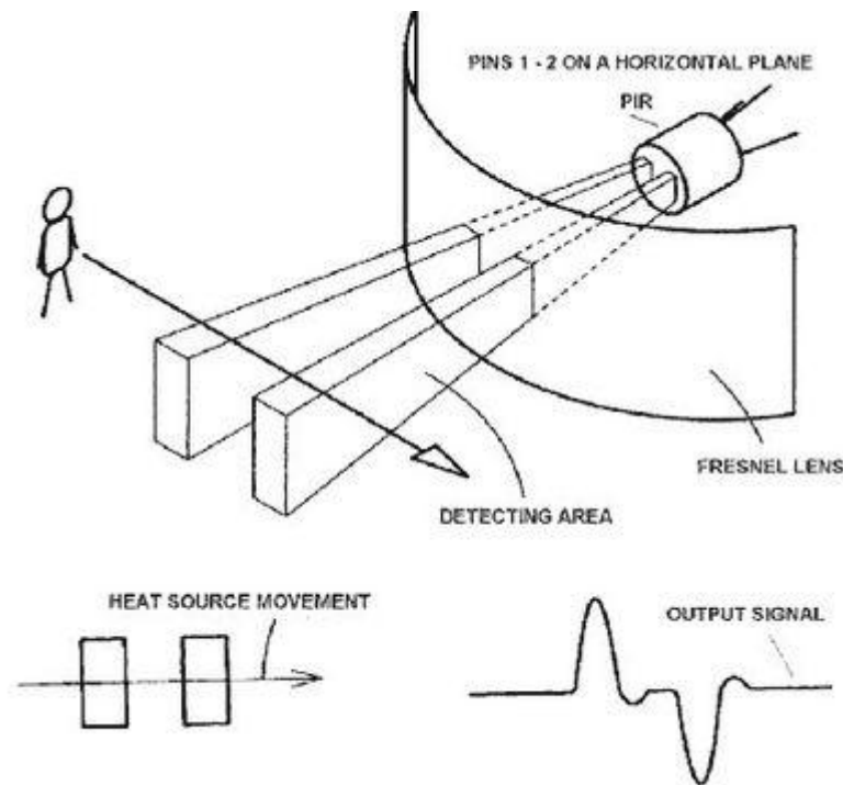
Figura 7: Diagrama del funcionamiento de un sensor PIR
