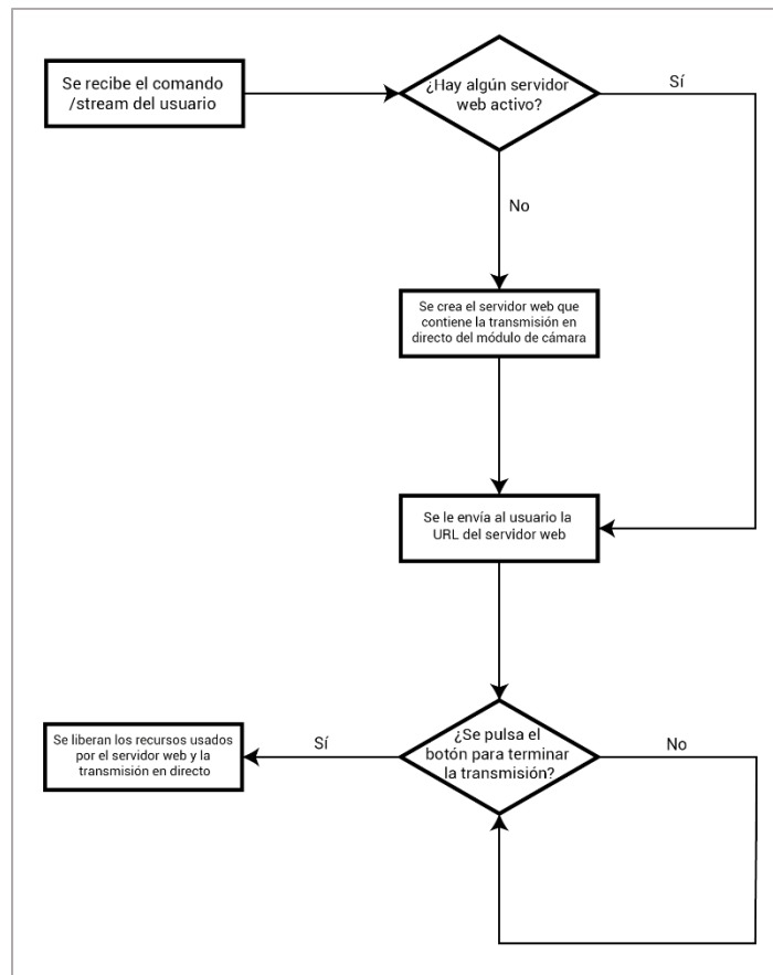
Figura 67: Flujograma del comando /stream
