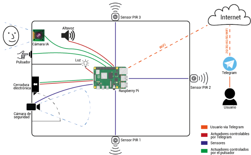
Figura 1: Esquema general del sistema de seguridad
