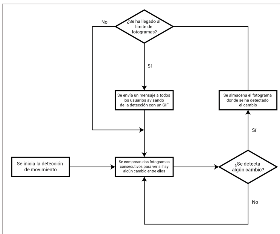
Figura 43: Flujograma del comando /detmo
