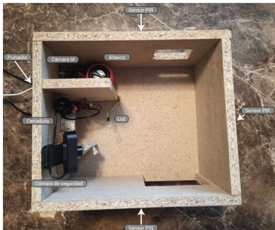
Figura 2: Vista de planta de la maqueta
