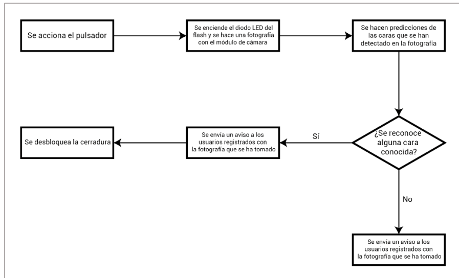
Figura 60: Flujograma para el reconocimiento facial
